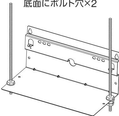
吊設置の場合 底面にボルト穴×2
