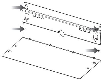
壁設置の場合 背面にビス穴×4
