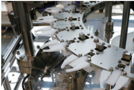
新規開発のネック搬送機構（特許出願中）
