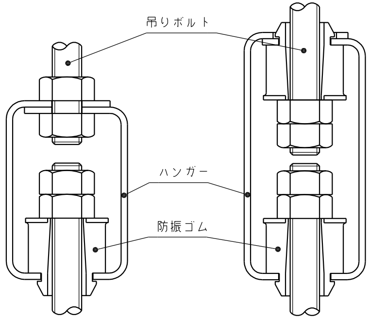
シングル取付け例
