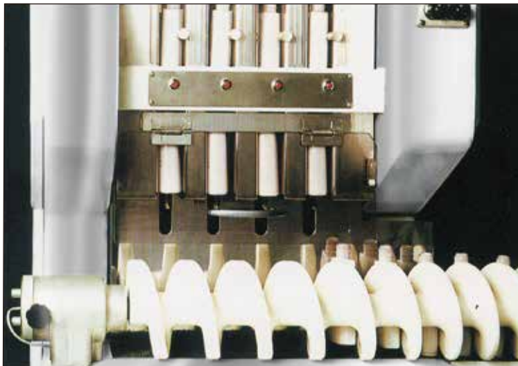
容器連続供給装置
